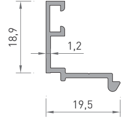
2027 KALIN CAM ÇİTASI TIRNAK ADAPTÖR 0.170 kg/mt
