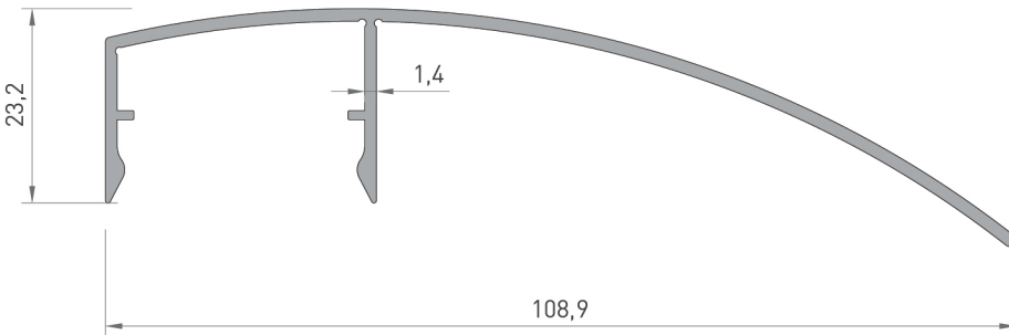
5322 MAFSALLI CEPHE KAPAK 0.640 kg/mt
