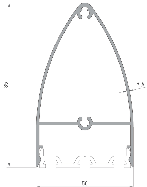
5313 BADEM KAPAK DÜŞEY - YATAY 0.995 kg/mt
