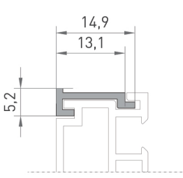
5290 KASET BANT TİJİ (ELOKSAL) 0.075 kg/mt
