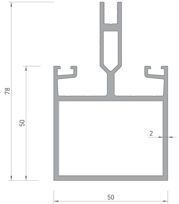
5007 DÜŞEY (YATAY) GRIYAJ 1.555 kg/mt Jx : 28.19 \text{ cm}^4 Jy : 15.93 \text{ cm}^4
