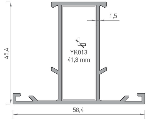
2202 DAR ORTA KAYIT PROFİLİ 0,770 kg/mt
