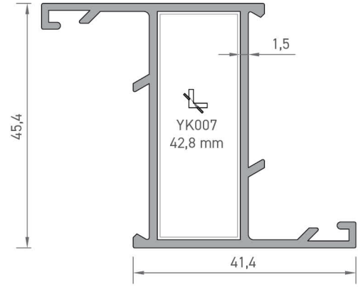
2201 DAR KANAT PROFİLİ 0,770 kg/mt
