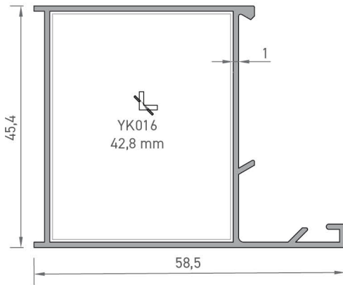
2183 GENİŞ KASA PROFİLİ 0,550 kg/mt
