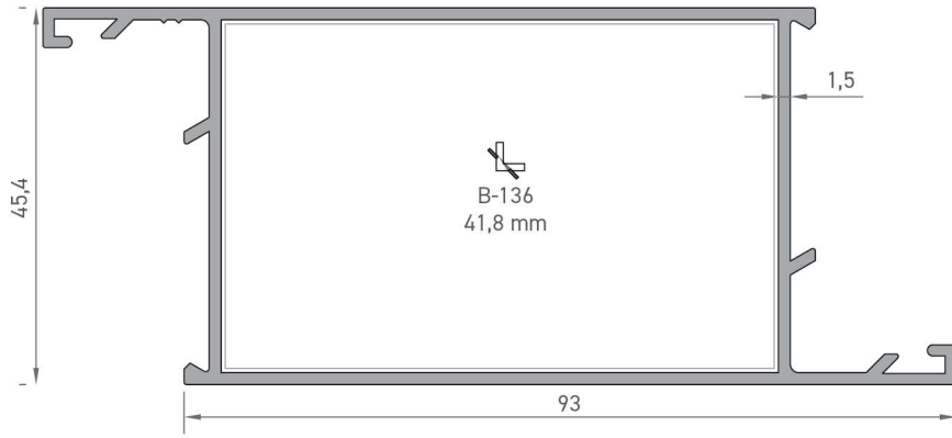
2198 BAZA KANAT PROFİLİ 1,165 kg/mt
