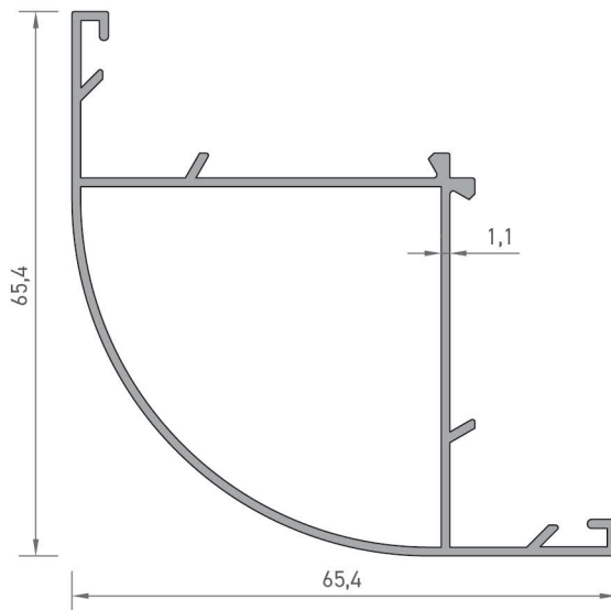
2172 OVAL KÖŞE PROFİLİ 0,680 kg/mt
