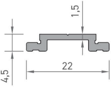
2640 TİJ ÇUBUK DIŞ PROFİLİ 0,130 kg/mt
