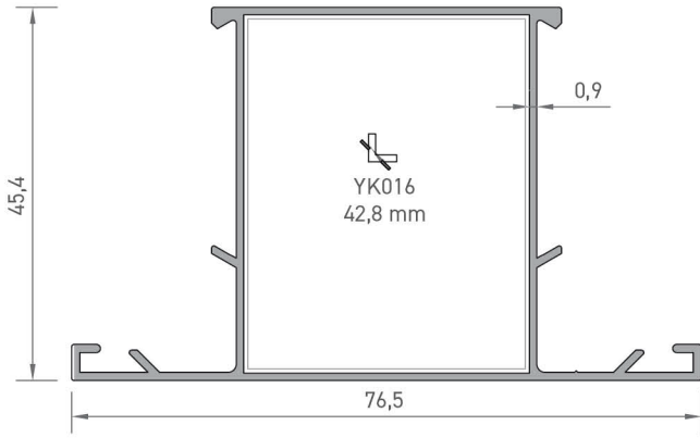
6095 GENİŞ ORTA KAYIT PROFİLİ 0,603 kg/mt
