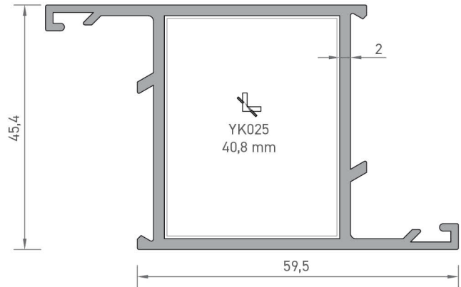
2187 GENİŞ KANAT PROFİLİ 1,165 kg/mt
