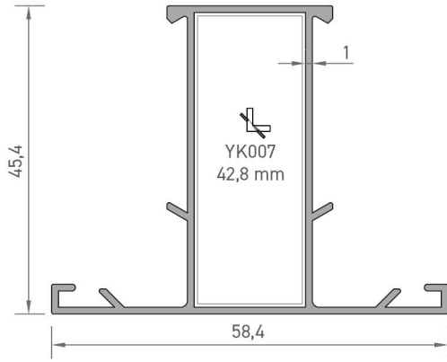
2179 DAR ORTA KAYIT PROFİLİ 0,550 kg/mt
