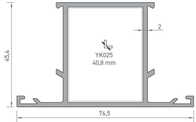
2186 GENİŞ ORTA KAYIT PROFİLİ 1,165 kg/mt
