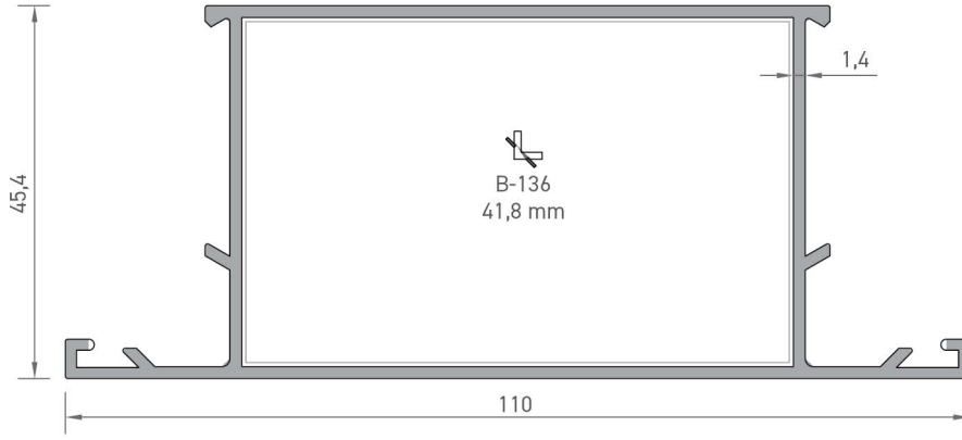
2207 BAZA ORTA KAYIT PROFİLİ 1,160 kg/mt
