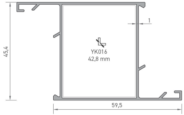
2181 GENİŞ KANAT PROFİLİ 0,645 kg/mt
