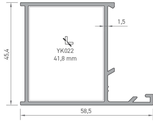
2206 GENİŞ KASA PROFİLİ 0,800 kg/mt
