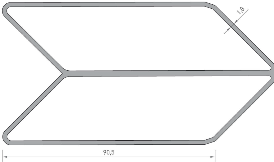
2109 ÇAVUŞ KÖŞE PROFİLİ 2,205 kg/mt
