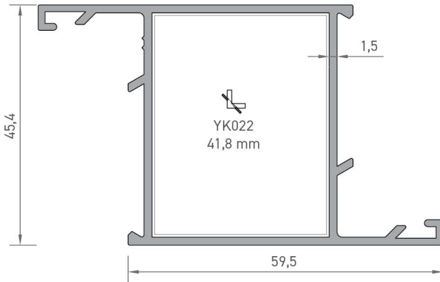
2204 GENİŞ KANAT PROFİLİ 0,925 kg/mt
