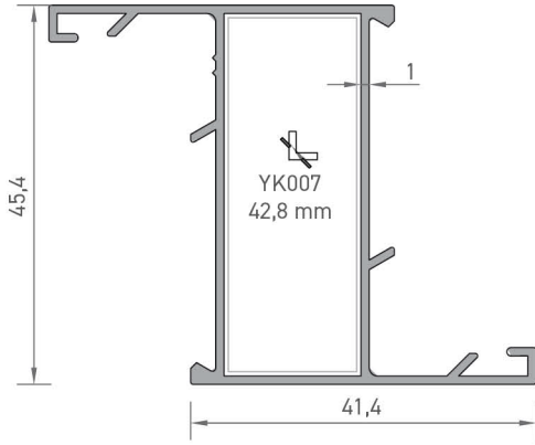
2178 DAR KANAT PROFİLİ 0,550 kg/mt
