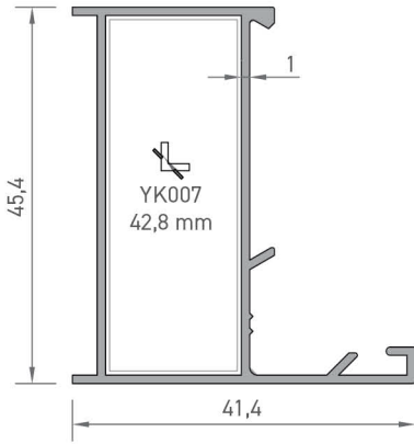
2180 DAR KASA PROFİLİ 0,460 kg/mt
