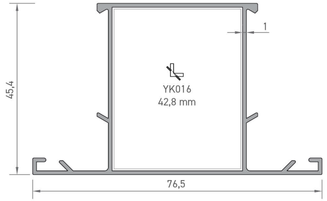
2182 GENİŞ ORTA KAYIT PROFİLİ 0,645 kg/mt
