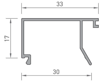
4178 TEK CAM ÇİTASI PROFİLİ 0,220 kg/mt
