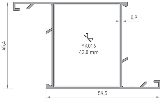
6096 GENİŞ KANAT PROFİLİ 0,603 kg/mt
