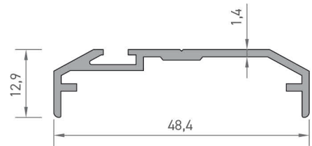
2175 ÇARPMA KAPI ADAPTÖR PROFİLİ 0,310 kg/mt
