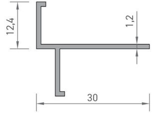
2530 FUGALI T 0,185 kg/mt
