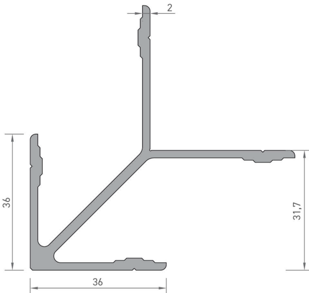
2151-B GENİŞ ÇAVUŞ KÖŞE BAĞLANTI PROFİLİ 1,180 kg/mt
