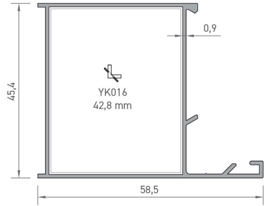
6094 GENİŞ KASA PROFİLİ 0,507 kg/mt
