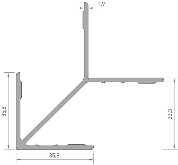
2151 GENİŞ ÇAVUŞ KÖŞE BAĞLANTI PROFİLİ 1,180 kg/mt
