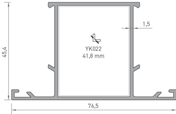
2205 GENİŞ ORTA KAYIT PROFİLİ 0,920 kg/mt
