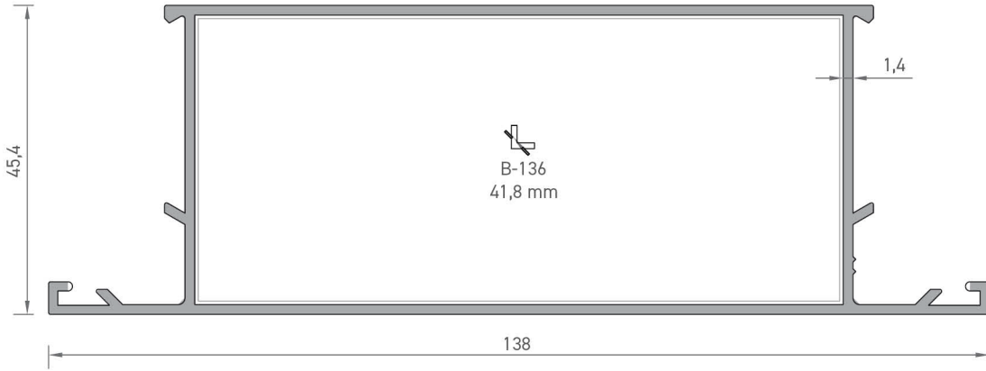
2110 BAZA ORTA KAYIT PROFİLİ 1,385 kg/mt
